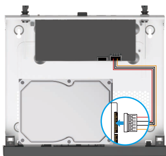
Připojení napájecího kabelu
