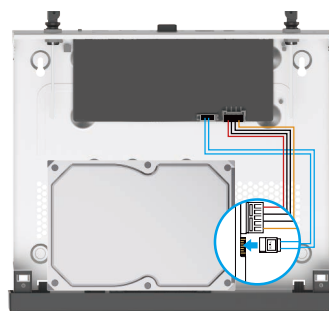
Připojení datového kabelu
